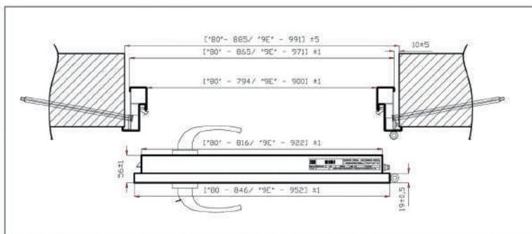
wymiary montażowe skrzydła wraz z ościeżnicą
