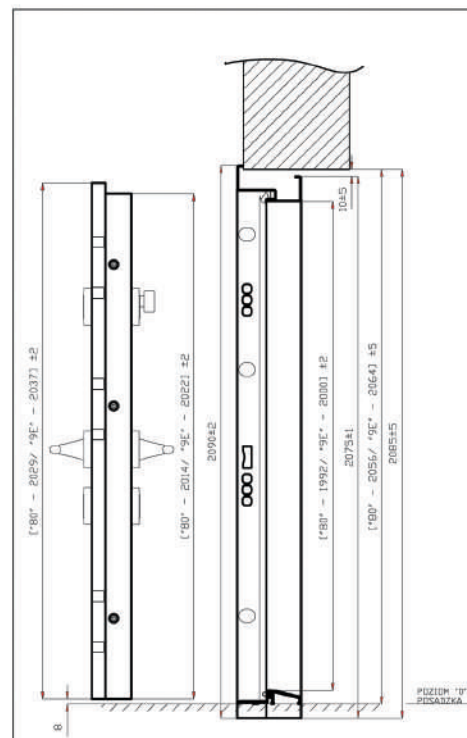
wymiary montażowe skrzydła względem posadzki
