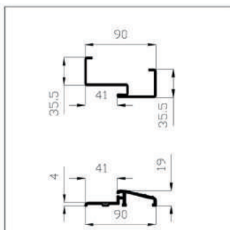
przekrój ościeżnicy i progu aluminiowego
